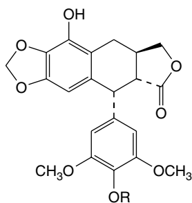
\beta -Peltatin, R = CH 3
