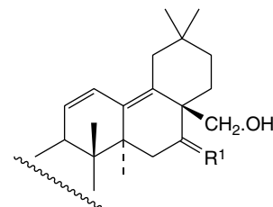
Saikosaponin b 2 , R^1 = \begin{matrix} \text{OH} \\ \diagup \\ \text{H} \end{matrix}
